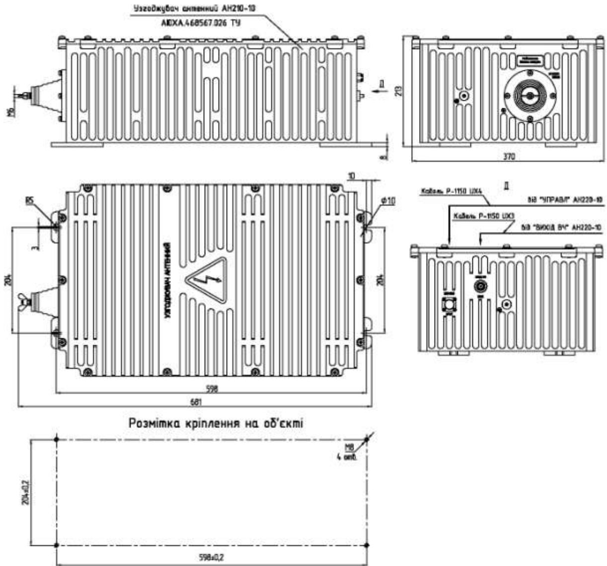
Рисунок 16 – Встановлення та з'єднання антенного узгоджувача
