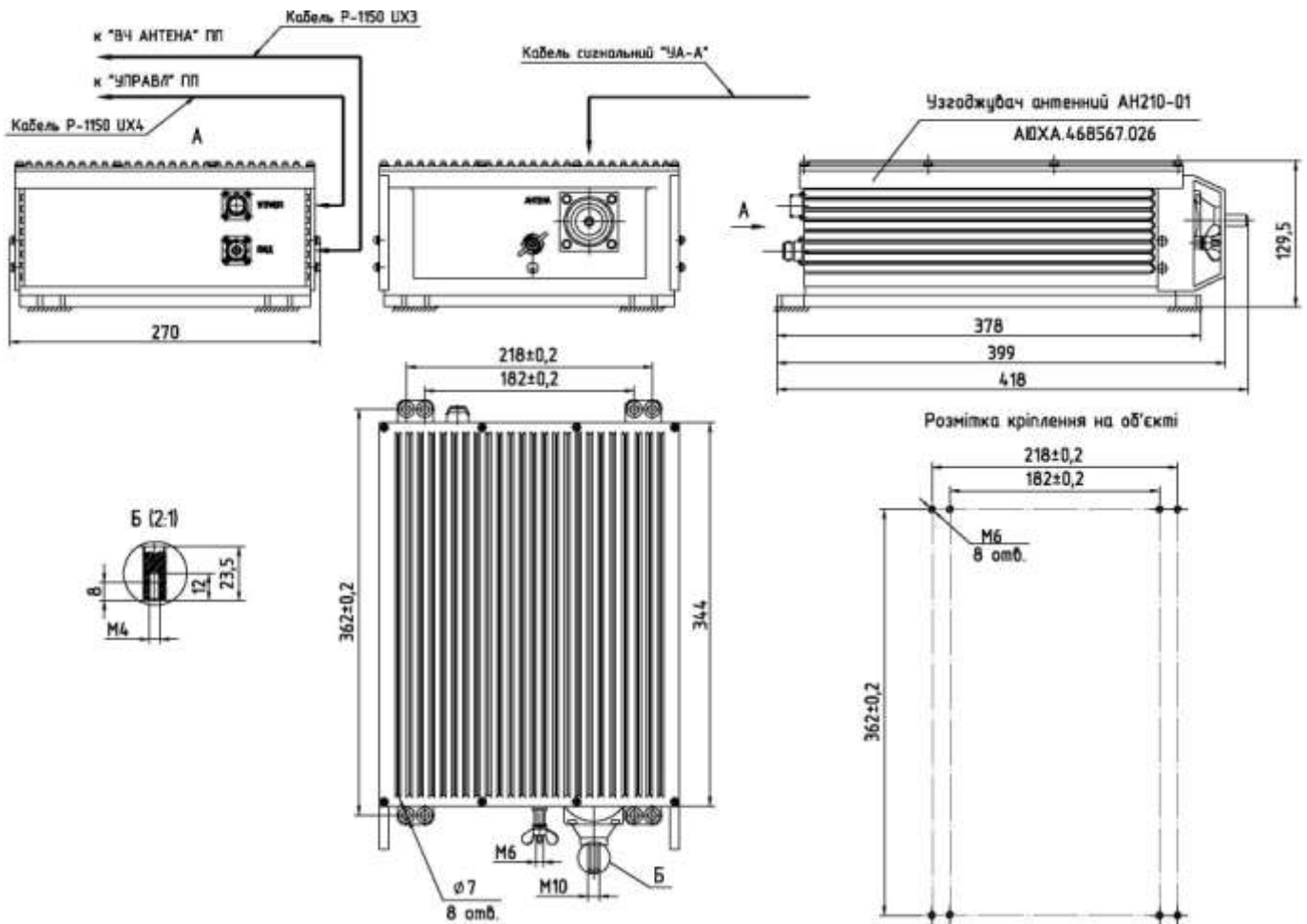
Рисунок 3 – Встановлення та з'єднання антенного узгоджувача
