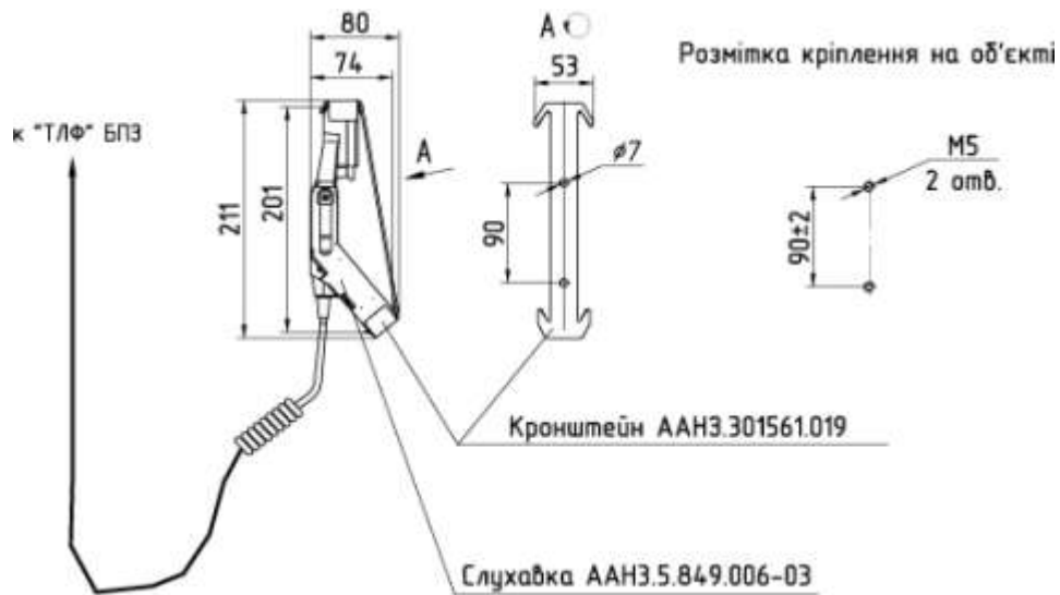
Рисунок 7 – Схема встановлення та підключення слухавки до радіостанції
