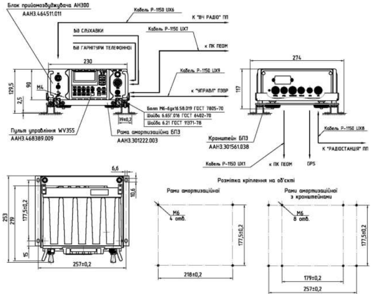
Рисунок 1 – Встановлення та з'єднання блоку прийомозбуджувача
