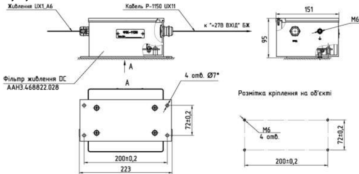
Рисунок 5 – Встановлення та з'єднання фільтра живлення DC
