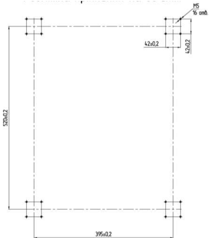
Рисунок 12 – Розмітка кріплення стійки монтажної радіопередавального пристрою на об'єкті
