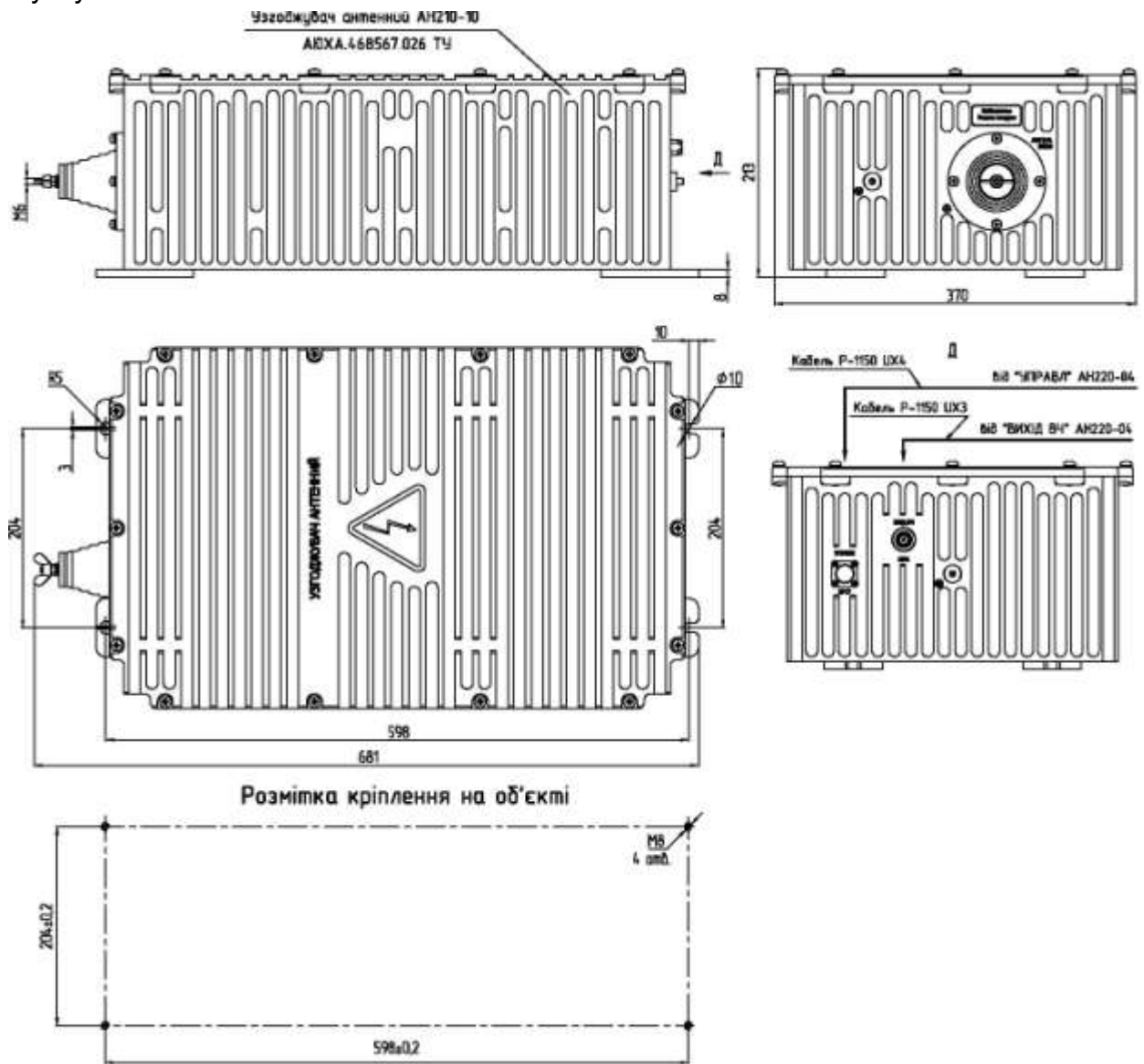
Рисунок 13 – Встановлення та з'єднання антенного узгоджувача
